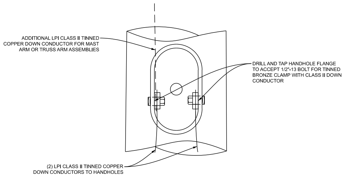
D DETAIL - POLE HANDHOLE N.T.S.
