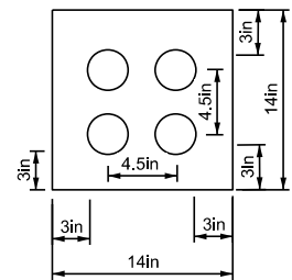
FOUR 3" CONDUIT
