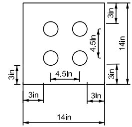
FOUR 2 1/2" CONDUIT
