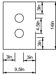
TWO 2 1/2" CONDUIT
