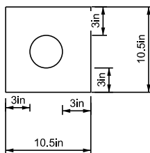
ONE 4" CONDUIT
