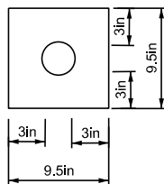
ONE 3" CONDUIT
