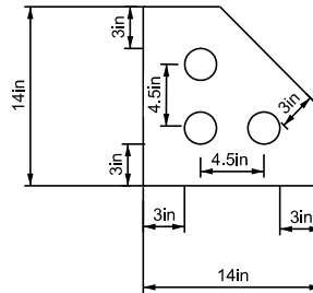
THREE 2 1/2" CONDUIT
