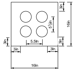
FOUR 4" CONDUIT
