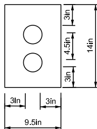
TWO 3" CONDUIT
