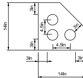
THREE 3" CONDUIT
