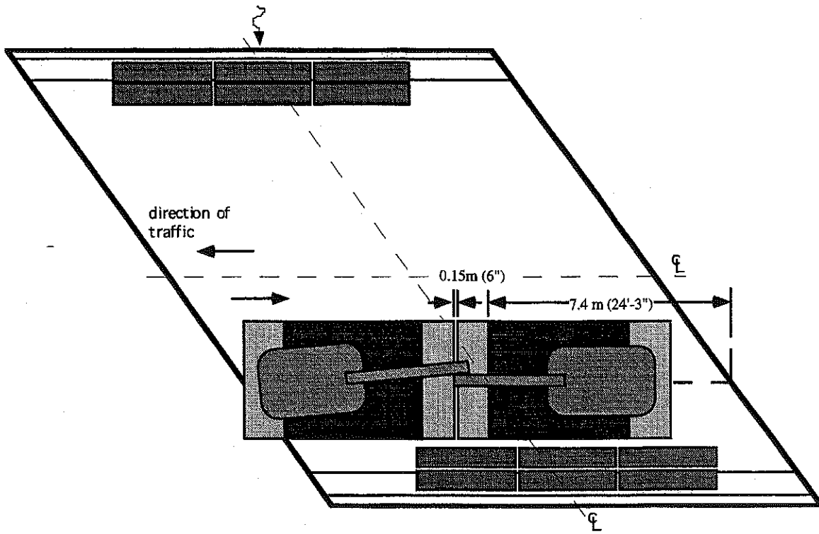
(d) Load Position 4 - Downstream Case.
