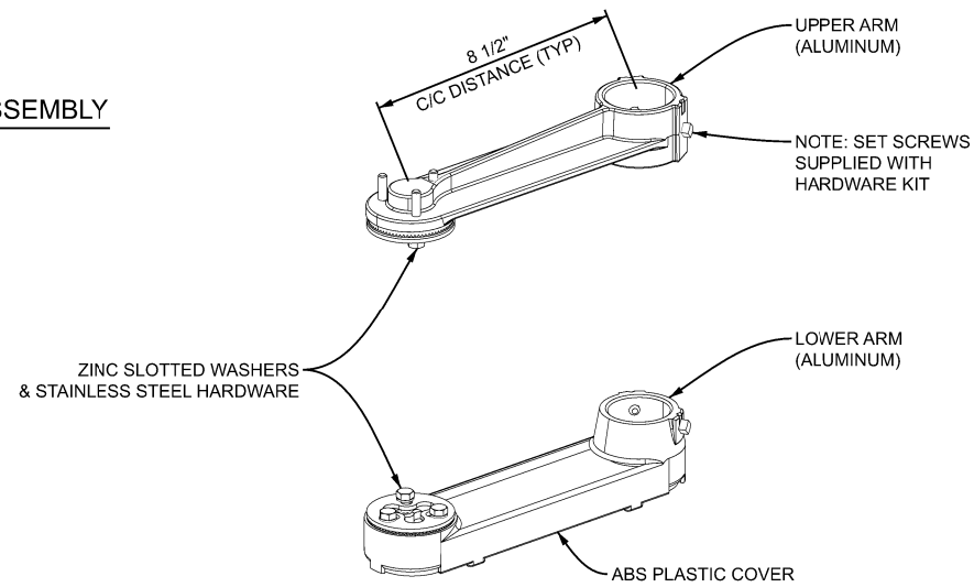
I DETAIL - 1-WAY BRACKET ARM ASSEMBLY N.T.S.
