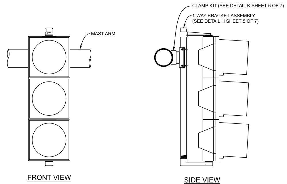
C DETAIL - 1W-3C N.T.S.
