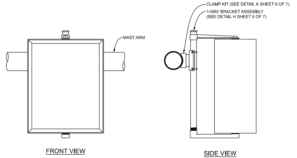
G DETAIL - 1W-CASE SIGN (24" X 30" SHOWN) N.T.S.
