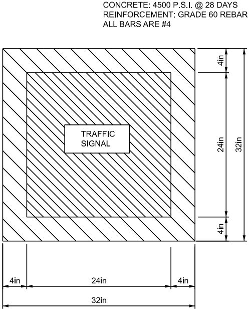
S DETAIL - PLAN VIEW N.T.S.
