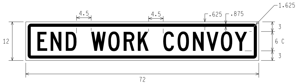
R5-18e END WORK CONVOY
