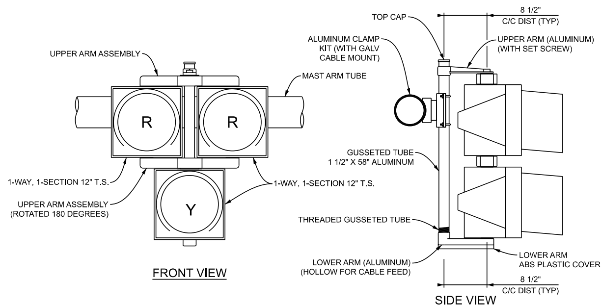
B DETAIL - MAST ARM DISPLAY N.T.S.
