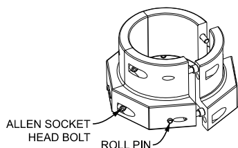
F COLLAR DETAIL - (OCTOGANAL BASE) N.T.S.
