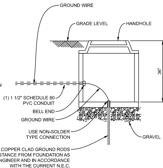
I DETAIL - HANDHOLE N.T.S.
