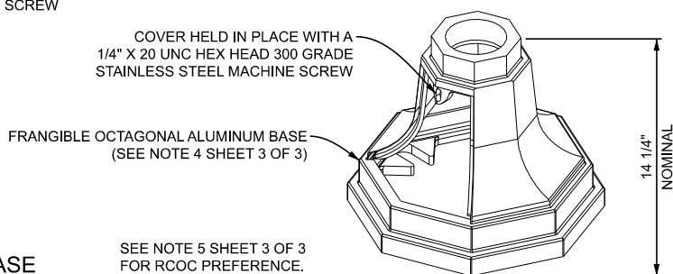
D DETAIL - OCTOGONAL BASE N.T.S.
