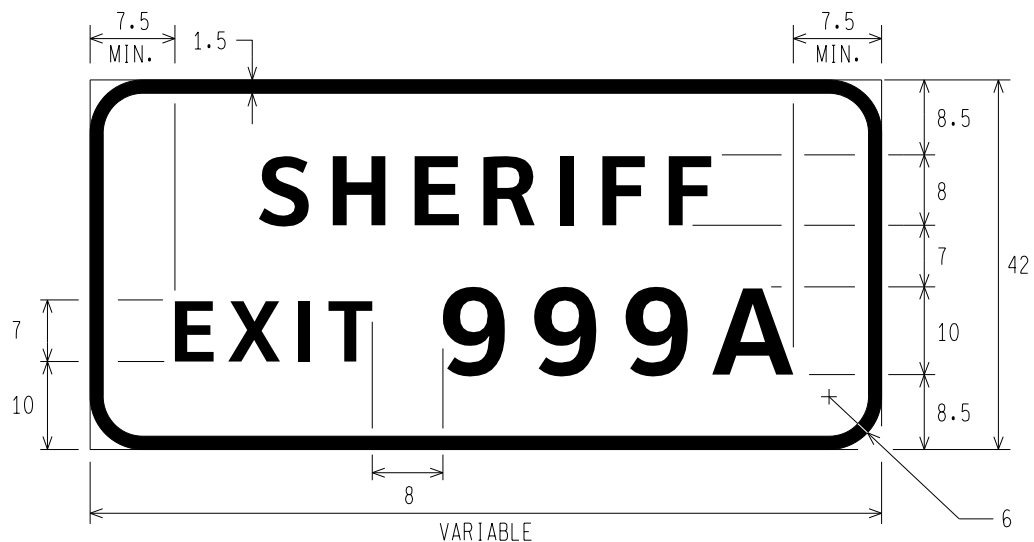
E11-9f SHERIFF EXIT
