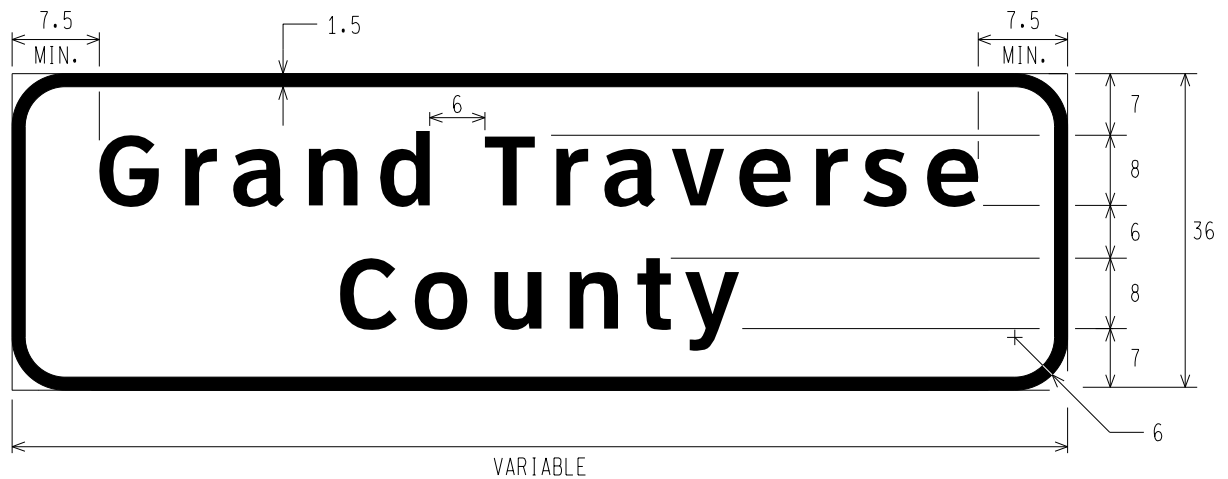
VARIABLE E11-6 COUNTY LIMIT
