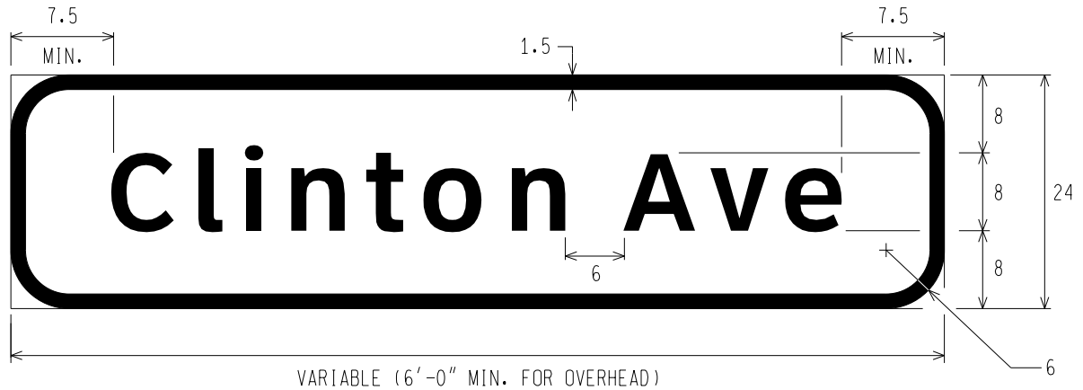
E11-3 ROAD NAME
