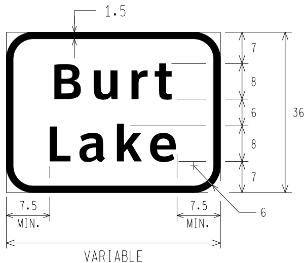
E11-8 LAKE IDENTIFIER
