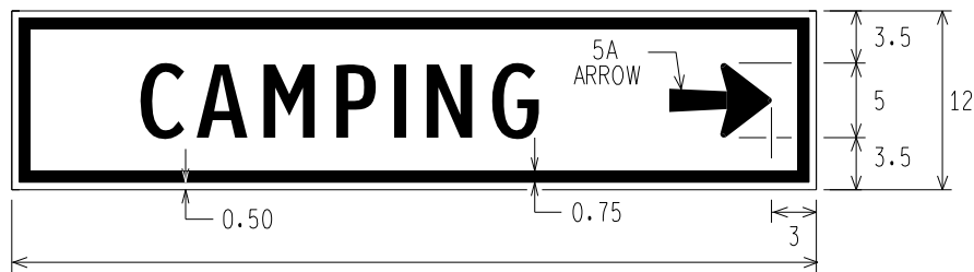
54 E11-15d [CAMPING] 2-W
