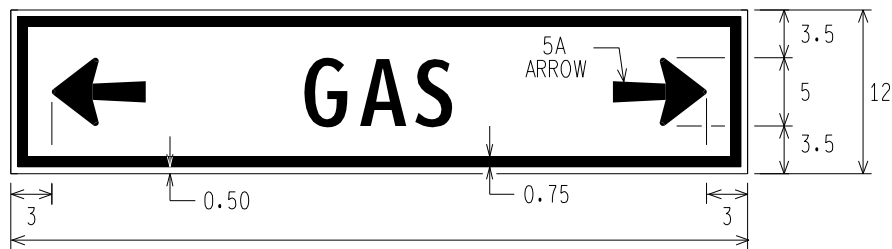
54 E11-15 [GAS] 2-W
