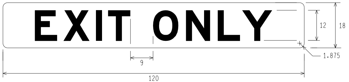
E11-1c EXIT ONLY
