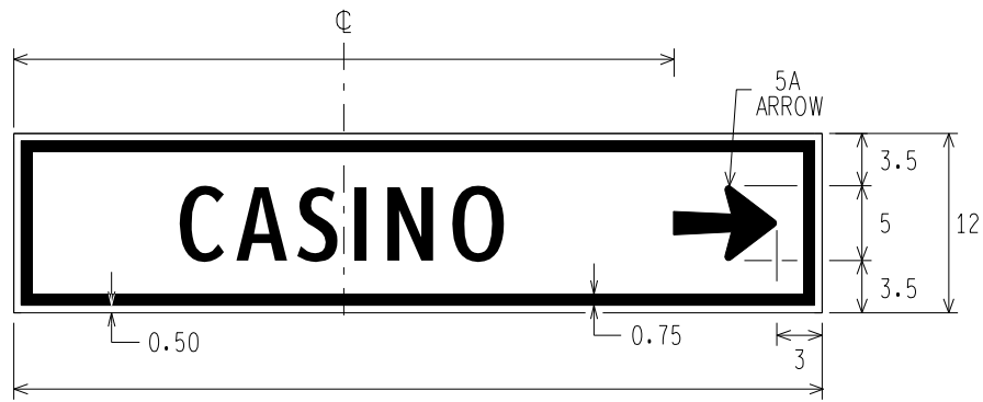
E11-15q [CASINO] 2-W
