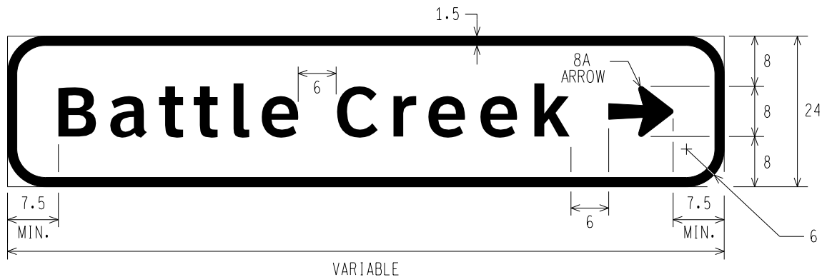
E11-4a DESTINATION ARROW
