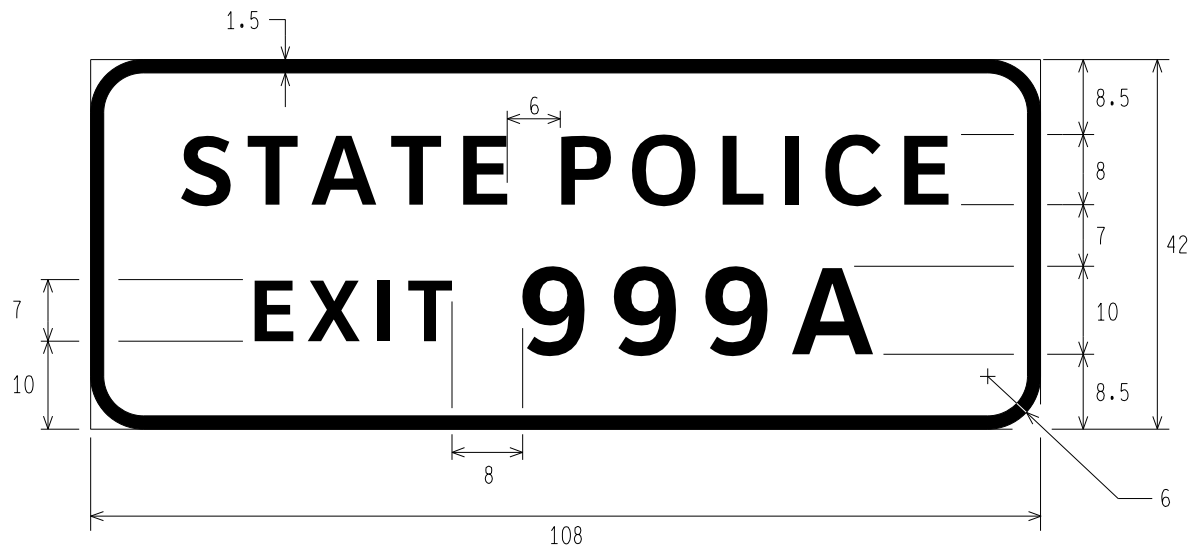
E11-9e STATE POLICE EXIT
