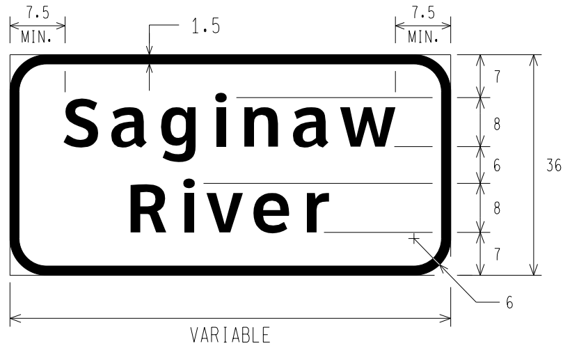
E11-7 RIVER/CREEK IDENTIFIER
