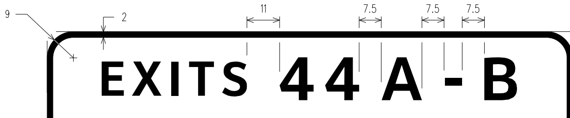
E1-5P EXIT PANEL DETAIL
