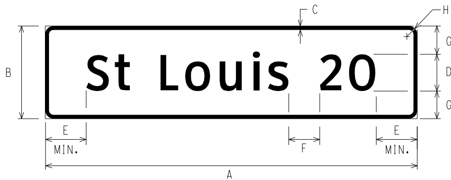
D2-1 DISTANCE (1 LINE)
