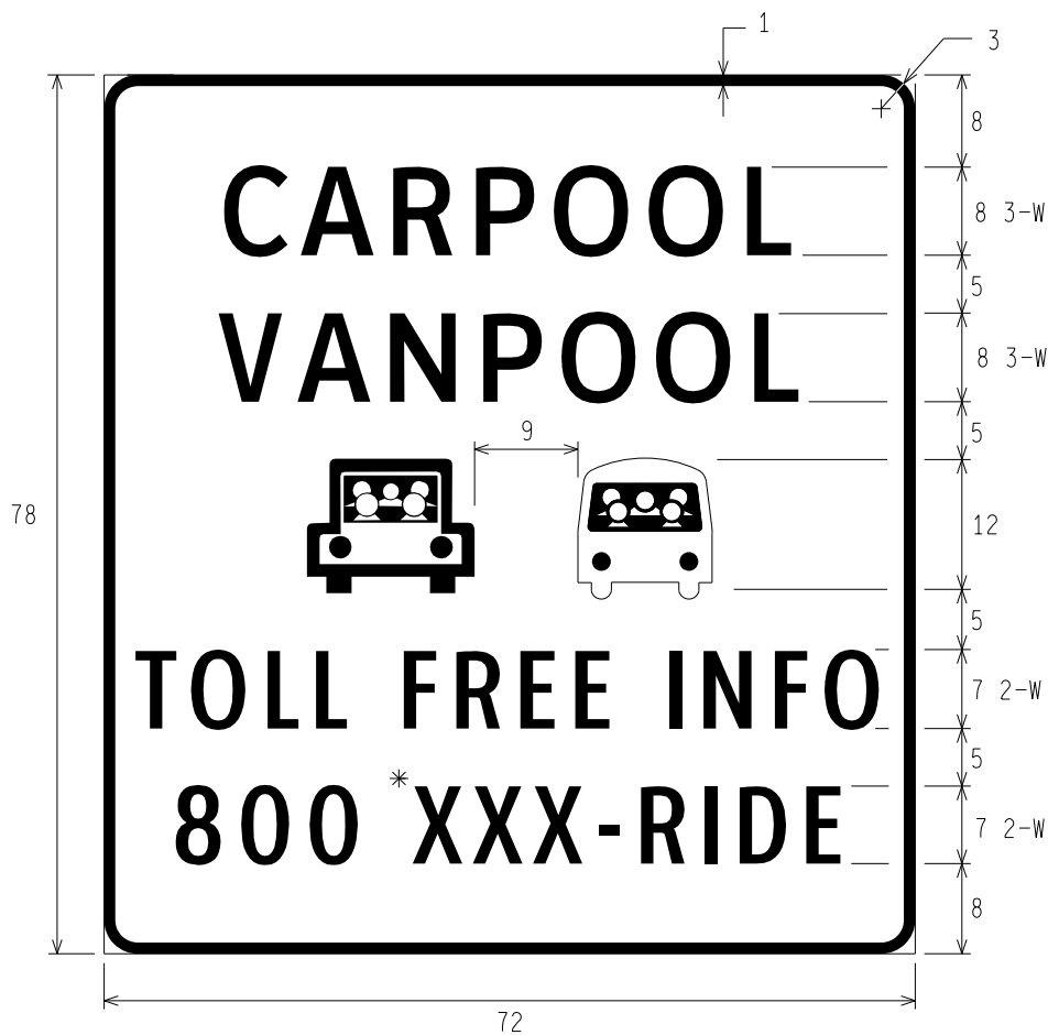
D12-2b CARPOOL VANPOOL INFORMATION
