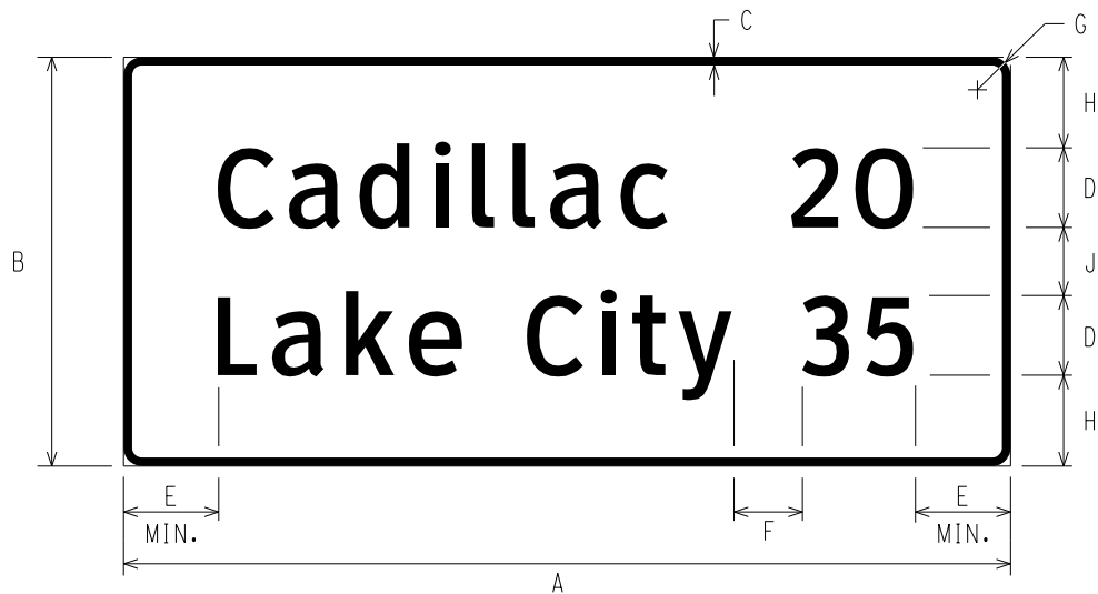
D2-2 DISTANCE (2 LINES)
