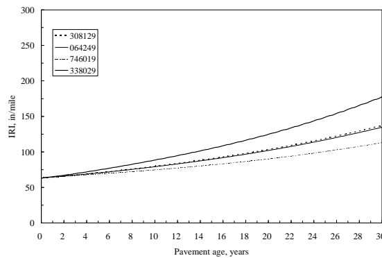
(c) IRI
