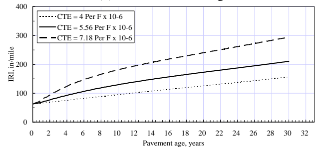
(c) IRI
