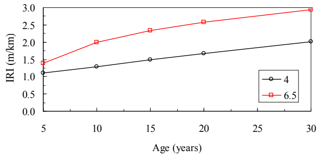
(d) Effect of CTE on IRI
