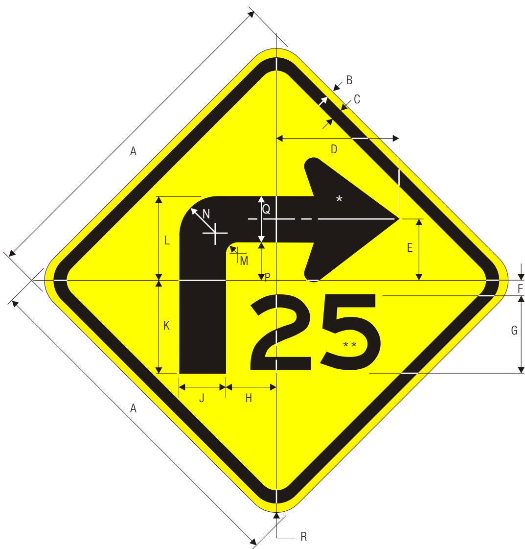
W1-1a R TURN
