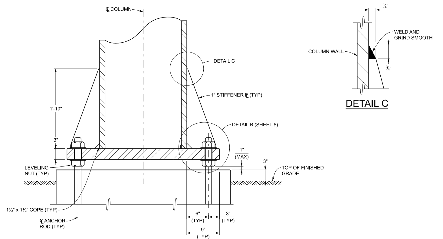
SECTION D-D
