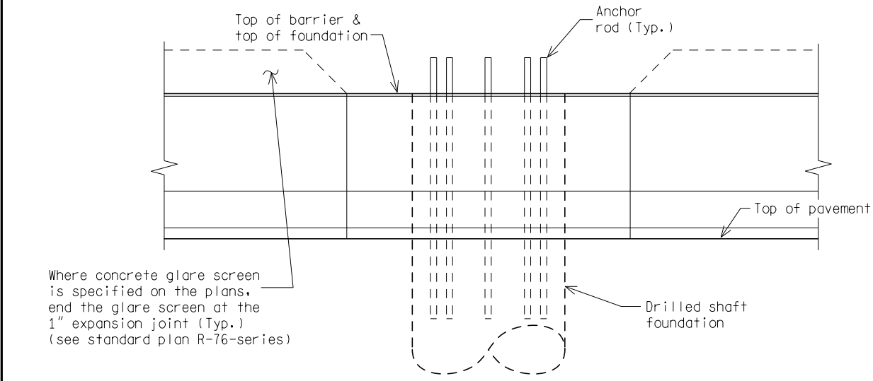
ELEVATION
