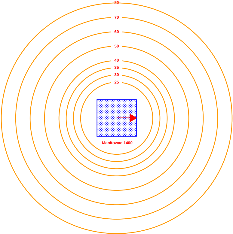
Manitowac 1400
